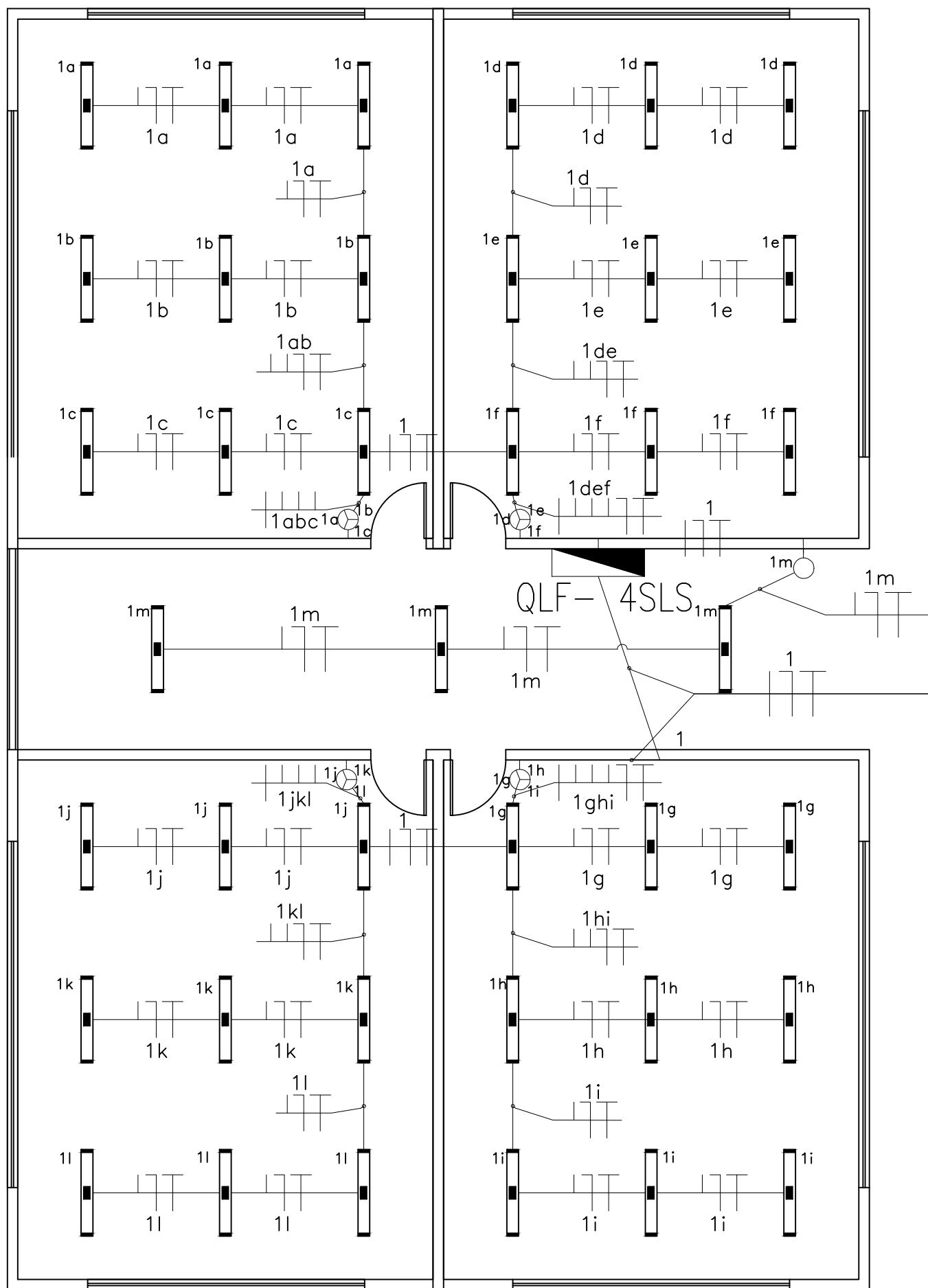
03 CIRCUITOS DE ILUMINAÇÃO ESCALA 1/75
