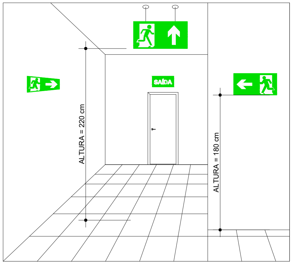
09 DET. FIXAÇÃO DAS PLACAS DE SINALIZAÇÃO DE EMERGÊNCIA SEM ESCALA
