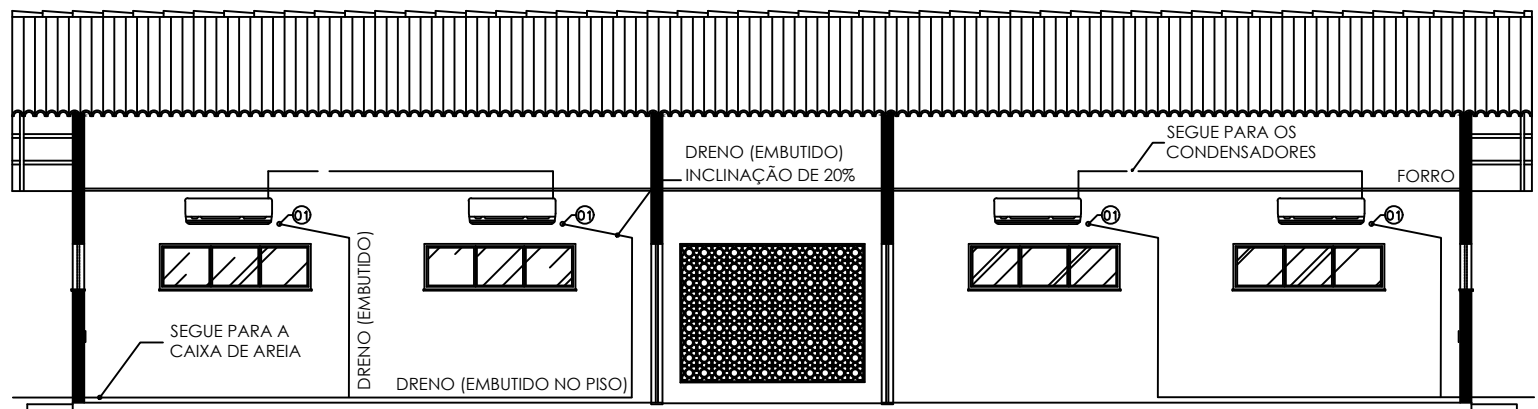
02 CORTE AA ESC 1/100
