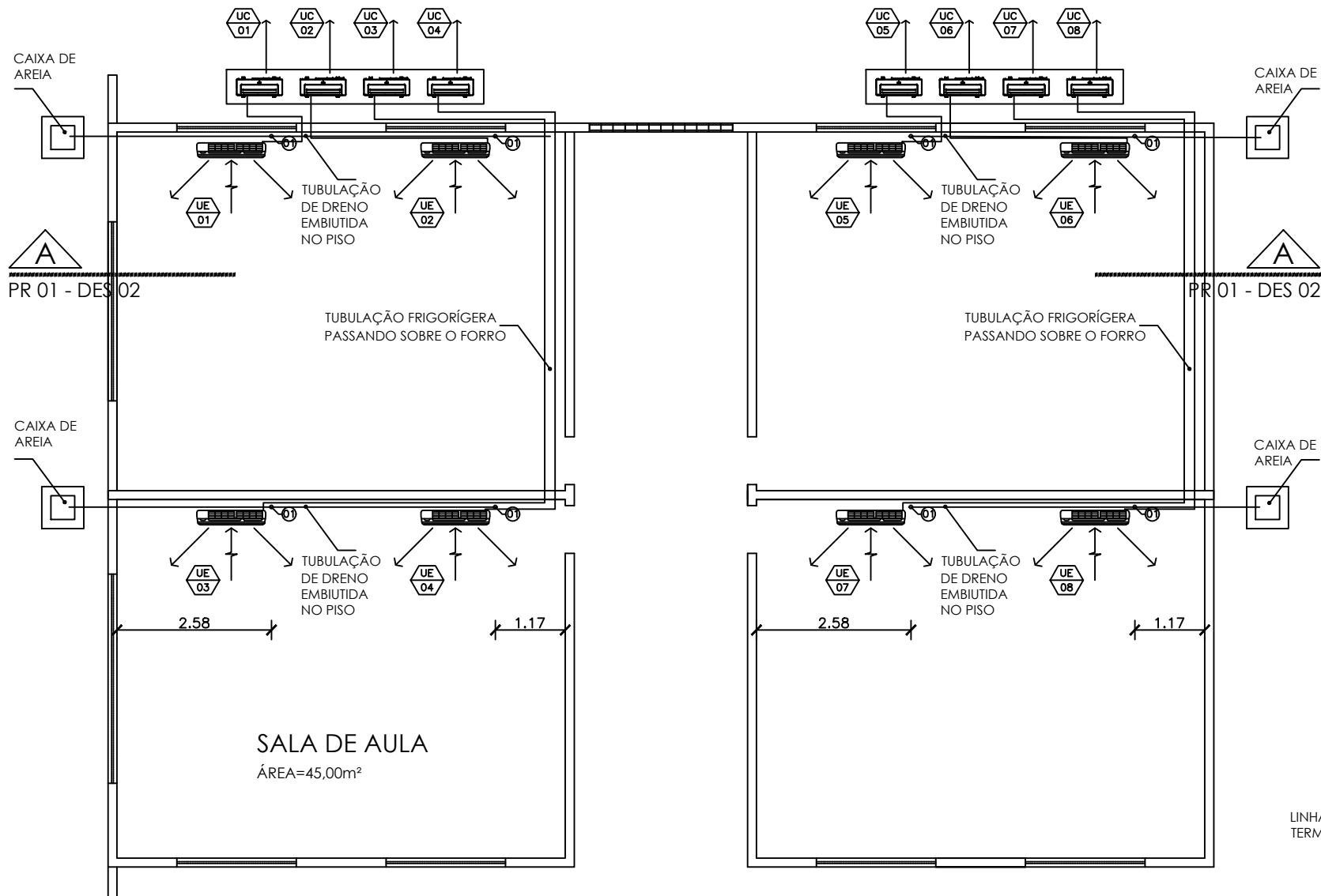
01 PLANTA BAIXA ESC 1/100
