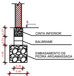
03 DETALHES EMBASAMENTO ESC 1/50
