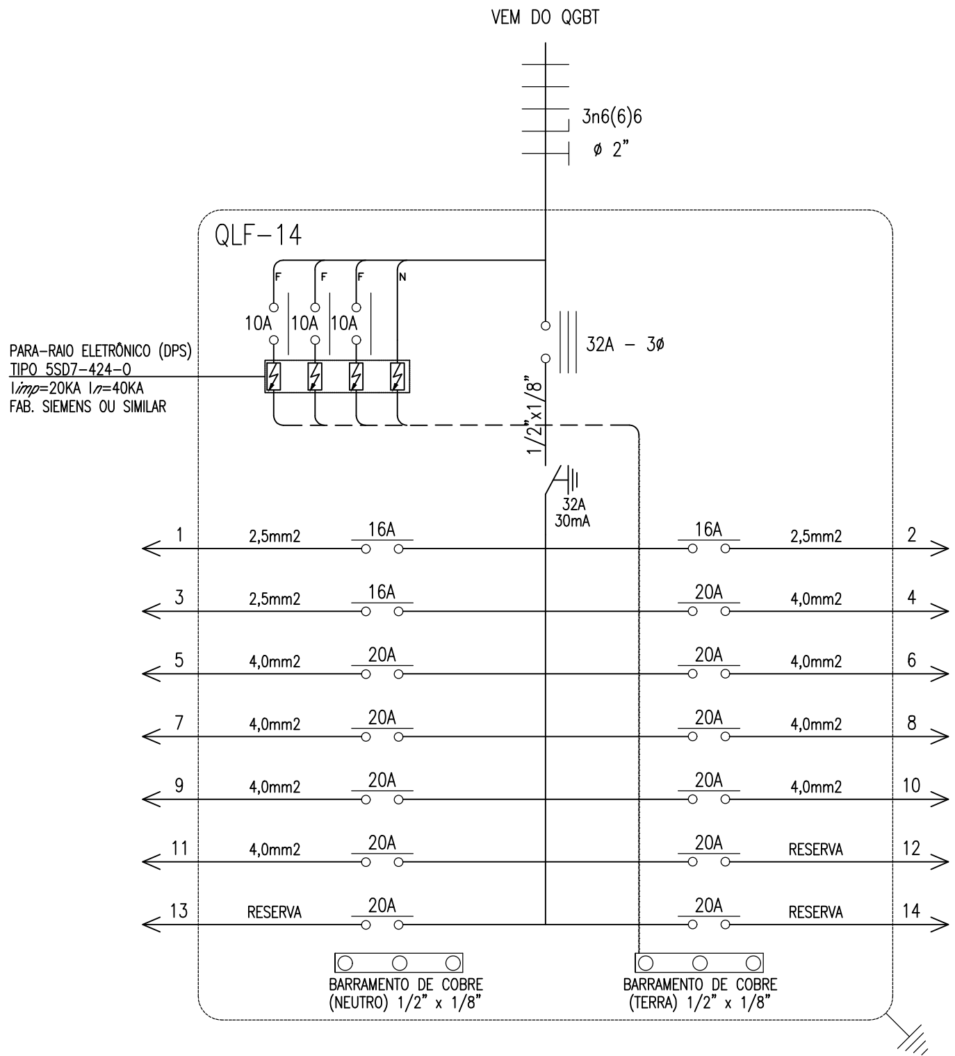
04 DIAGRAMA UNIFILAR SEM ESCALA
