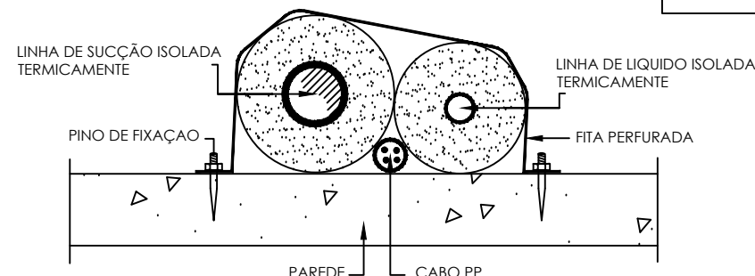
03 INTERLIGAÇÃO ENTRE UNIDADES SEM ESCALA
