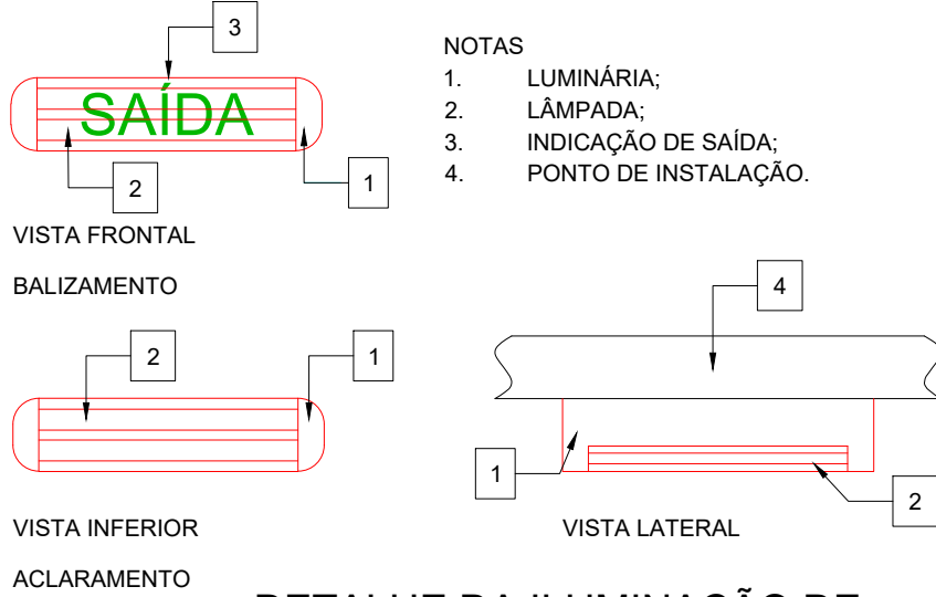
11 DETALHE DA ILUMINAÇÃO DE EMERGÊNCIA SEM ESCALA
