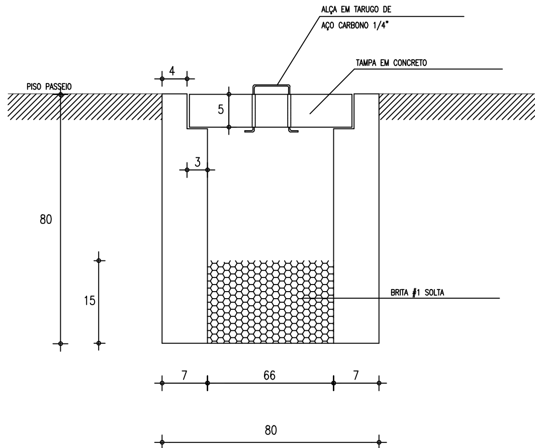
06 DETALHE DE CAIXA DE PASSAGEM SEM ESCALA
