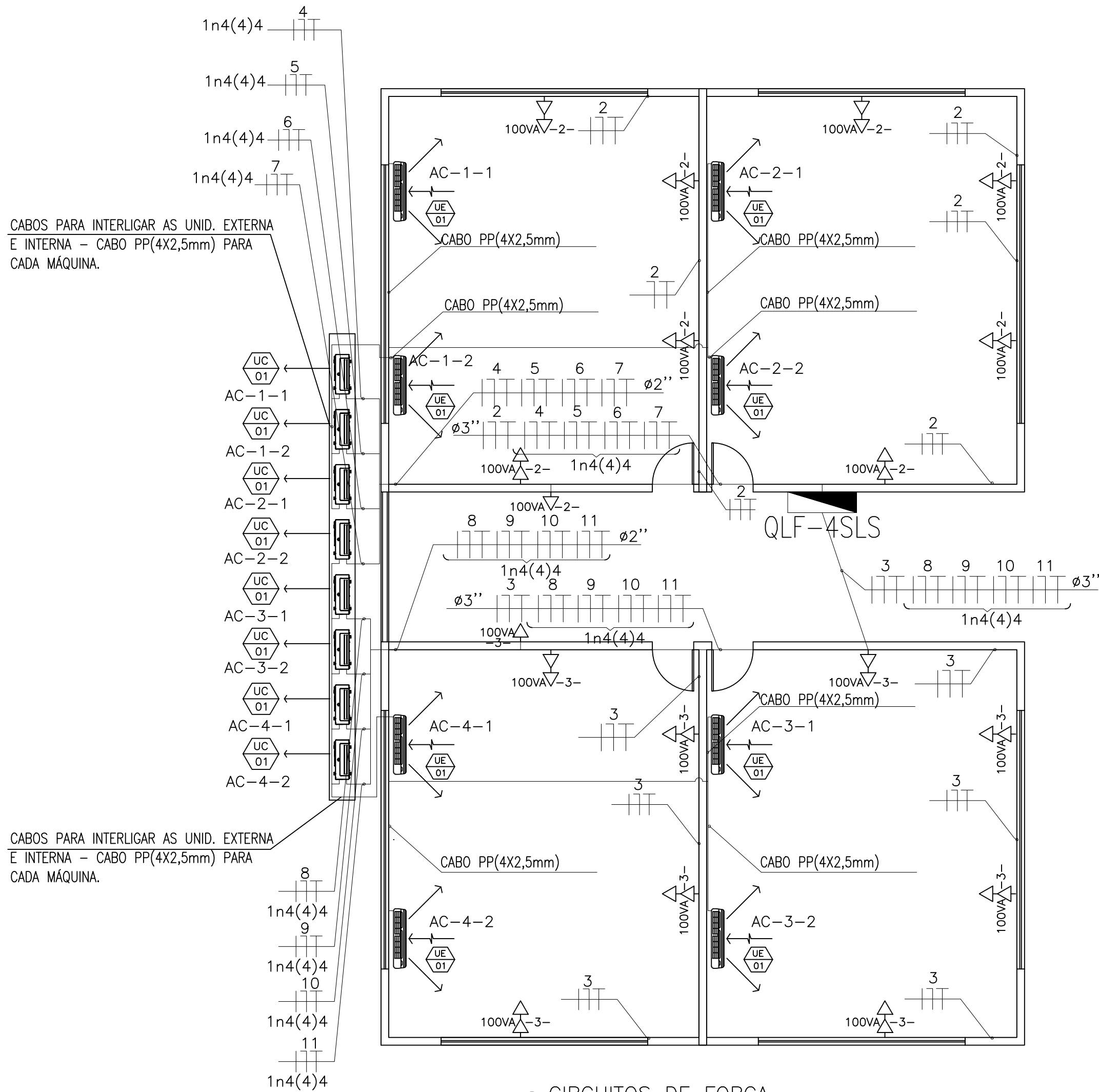
02 CIRCUITOS DE FORÇA ESCALA 1/75
