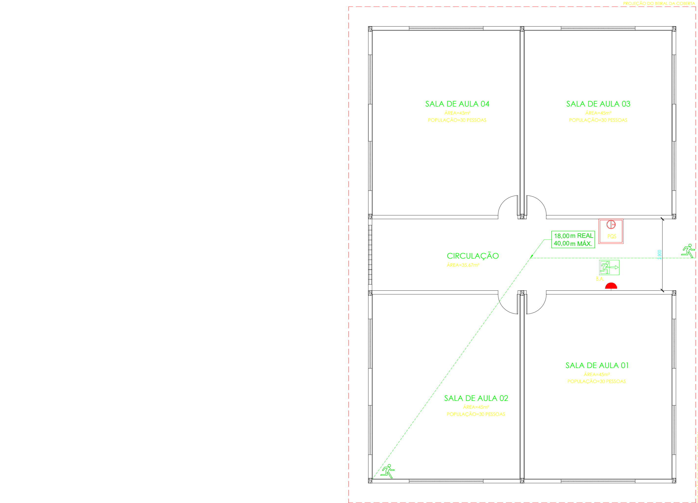
01 PLANTA BAIXA - SALAS DE AULA ESC 1/75
