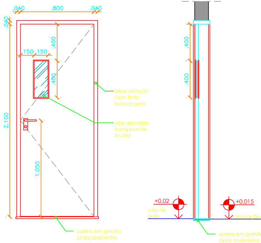
03 VISTA PORTA ESC 1/25
