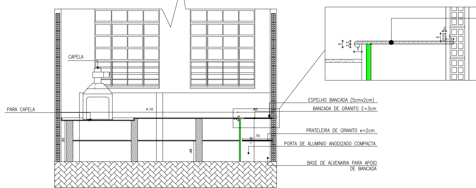
04 CORTE B/B ESCALA: 1/50
