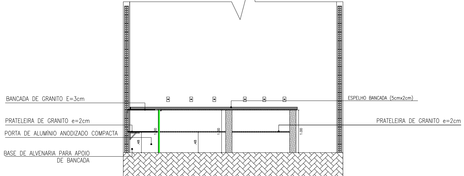
05 CORTE C/C ESCALA: 1/50
