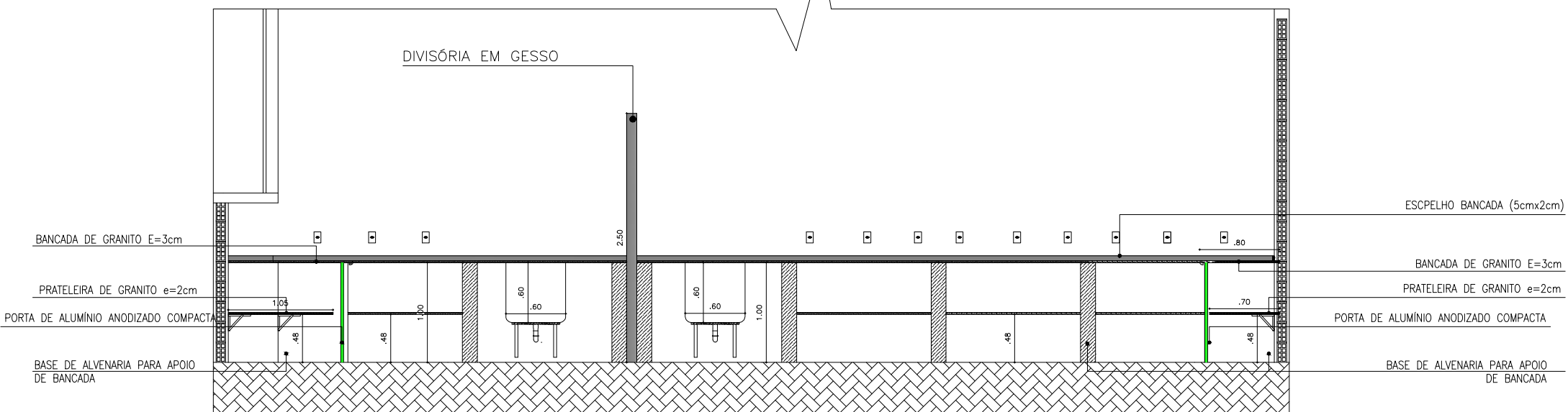
03 CORTE A/A ESCALA: 1/50
